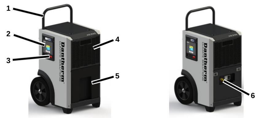
Fig. 1: Produktübersicht Vorderansicht
